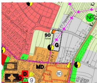
13. Flächennutzungsplan-Änderung 1:5000
